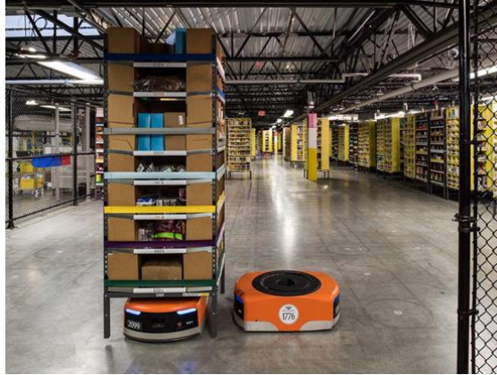
图3 亚马逊物流仓库中的机器人
